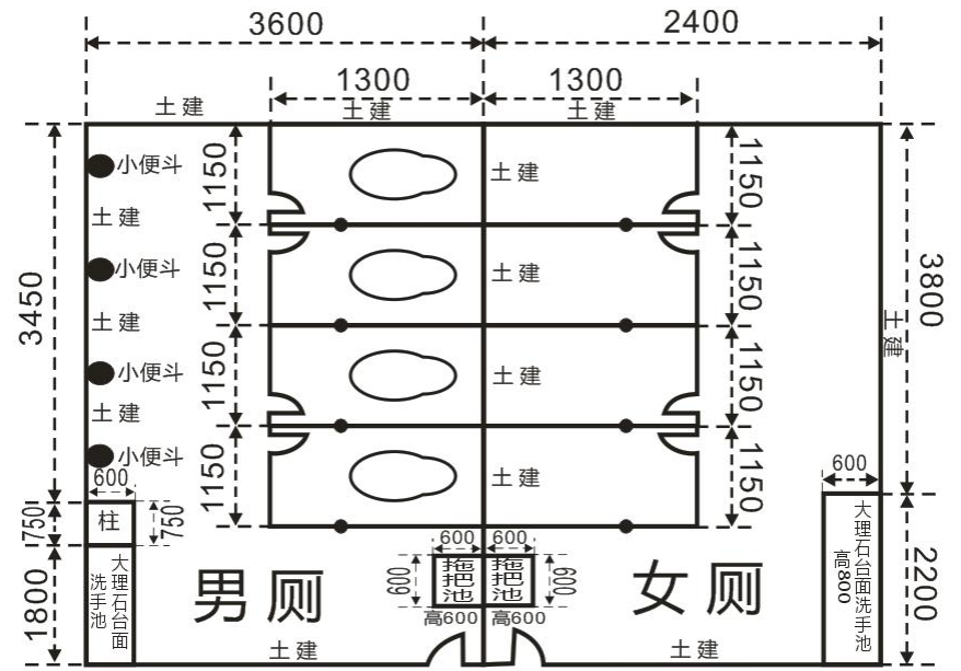
综合楼门诊二楼卫生间平面图二
