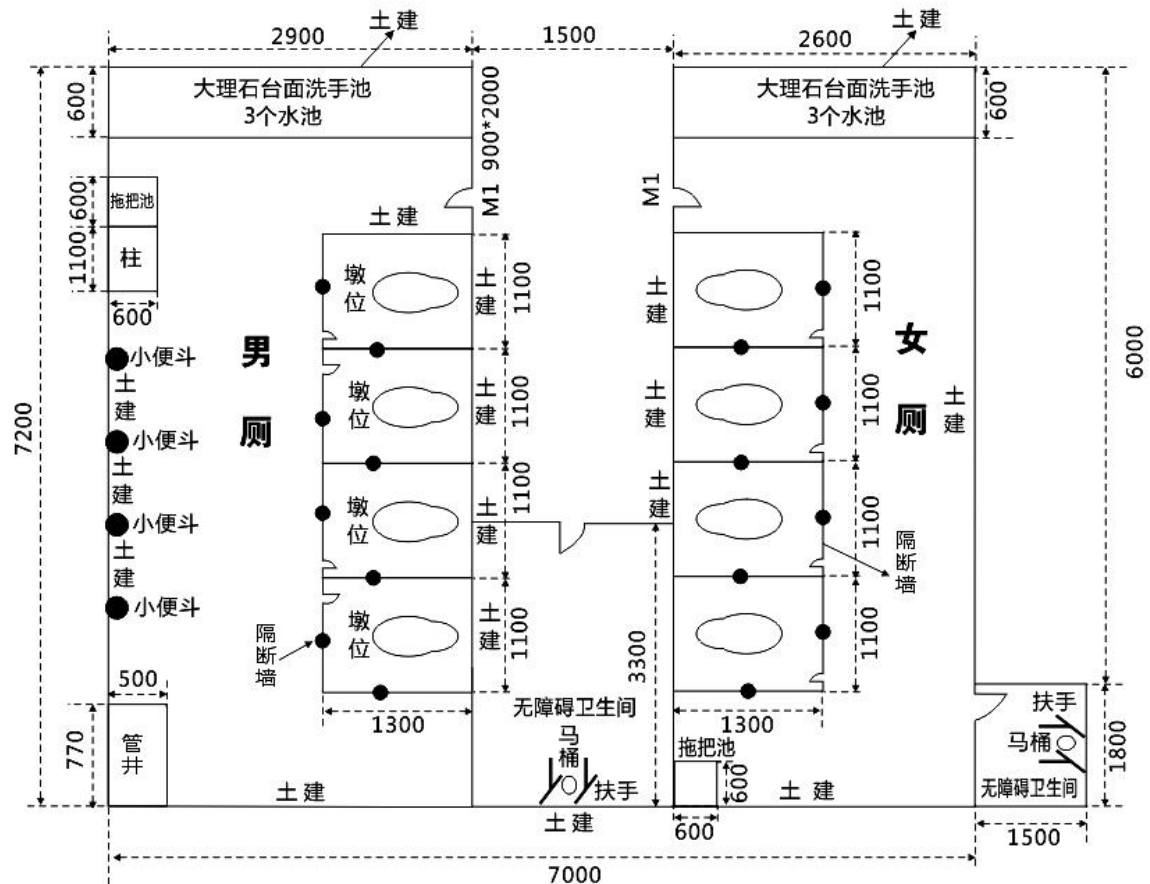
综合楼门诊三楼卫生间平面图
